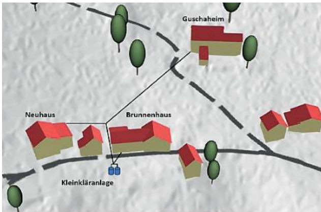
Situationsplan geplantes Abwasserleitungsnetz, Kleinkläranlage
